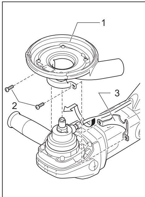
► 1. Couvercle de la meule diamantée à moyeu déporté 2. Vis 3. Collier d'installation
