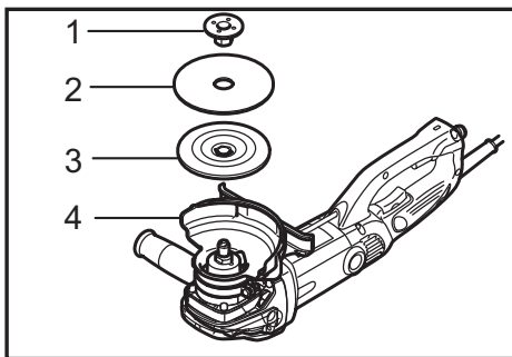
► 1. Contre-écrou 2. Disque abrasif 3. Plateau de caoutchouc 4. Couvercle à poussière 125 mm
