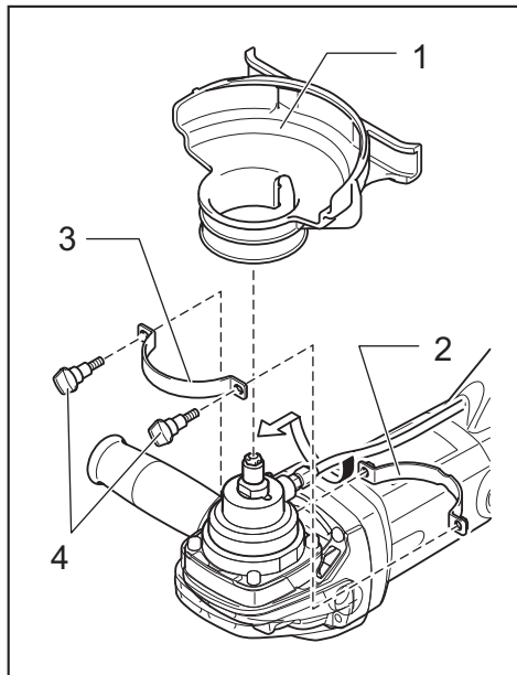
► 1. Couvercle à poussière 125 mm 2. Partie A du collier du couvercle à poussière 3. Partie B du collier du couvercle à poussière 4. Vis
